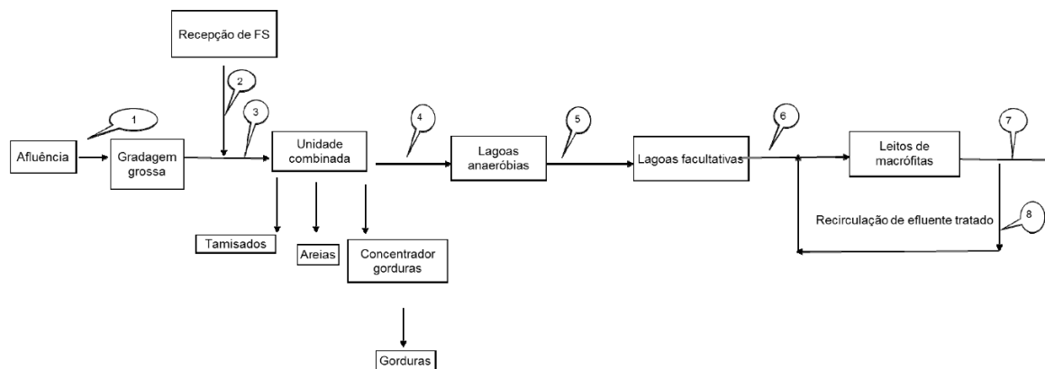
FIGURA 1 – DIAGRAMA SIMPLIFICADO DO PROCESSO DE TRATAMENTO
